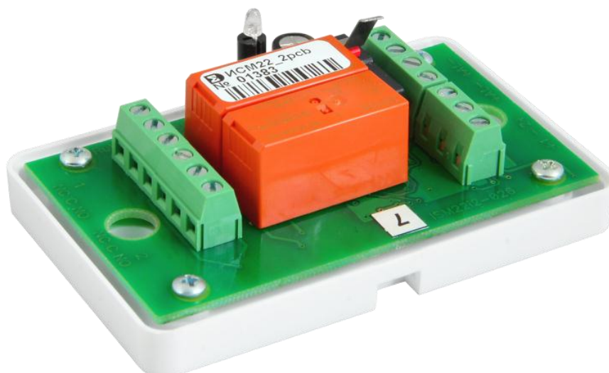
Рис. 1 Внешний вид ИСМ со снятой крышкой
