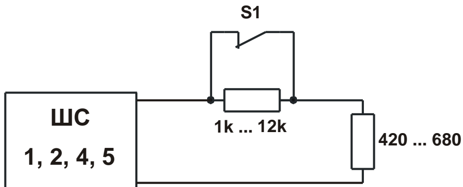
Рис. 6 Последовательное подключение 1 извещателя с НЗ контактами
