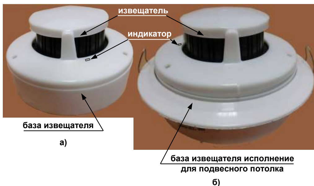
Рисунок 2 – Варианты исполнения АЗДПИ: а – извещатель с базой; б – извещатель с базой для подвесного потолка
