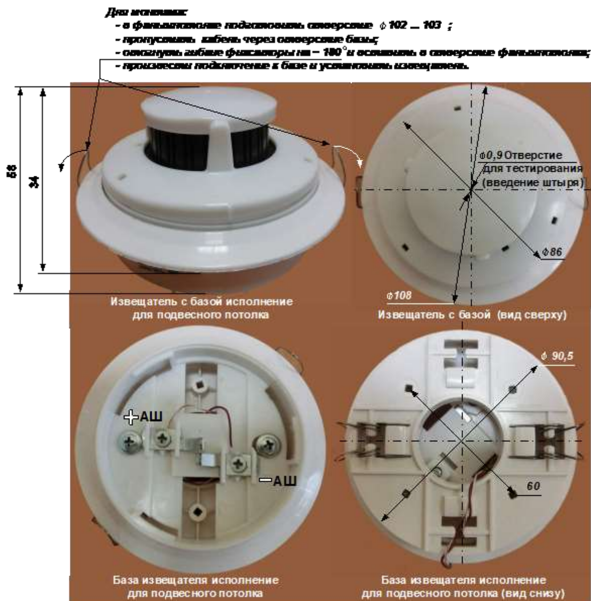
Рисунок 4 – АЗДПИ с базой для подвесного потолка. Габаритные и присоединительные размеры
