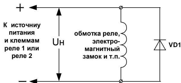
Рис. 7 Подключение индуктивной нагрузки(замок) к клеммам реле КД2
