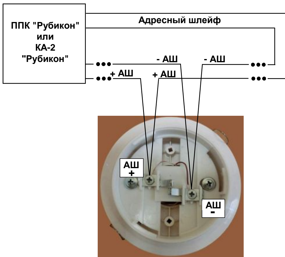
Рис. 4 Подключение АТИ
