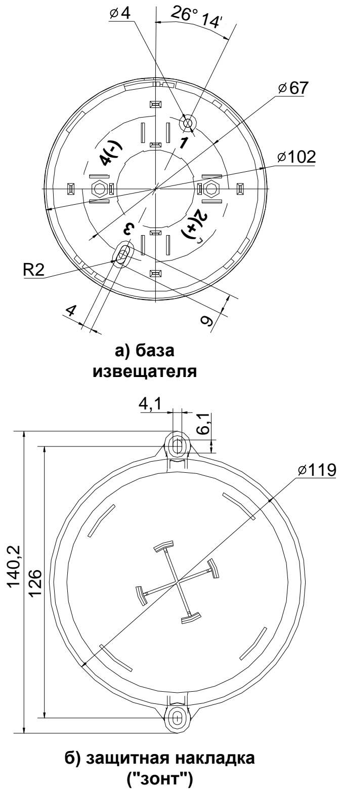
Рис. 3 А2ДПИ. Габаритные и присоединительные размеры базы и защитной накладки "Зонт"
