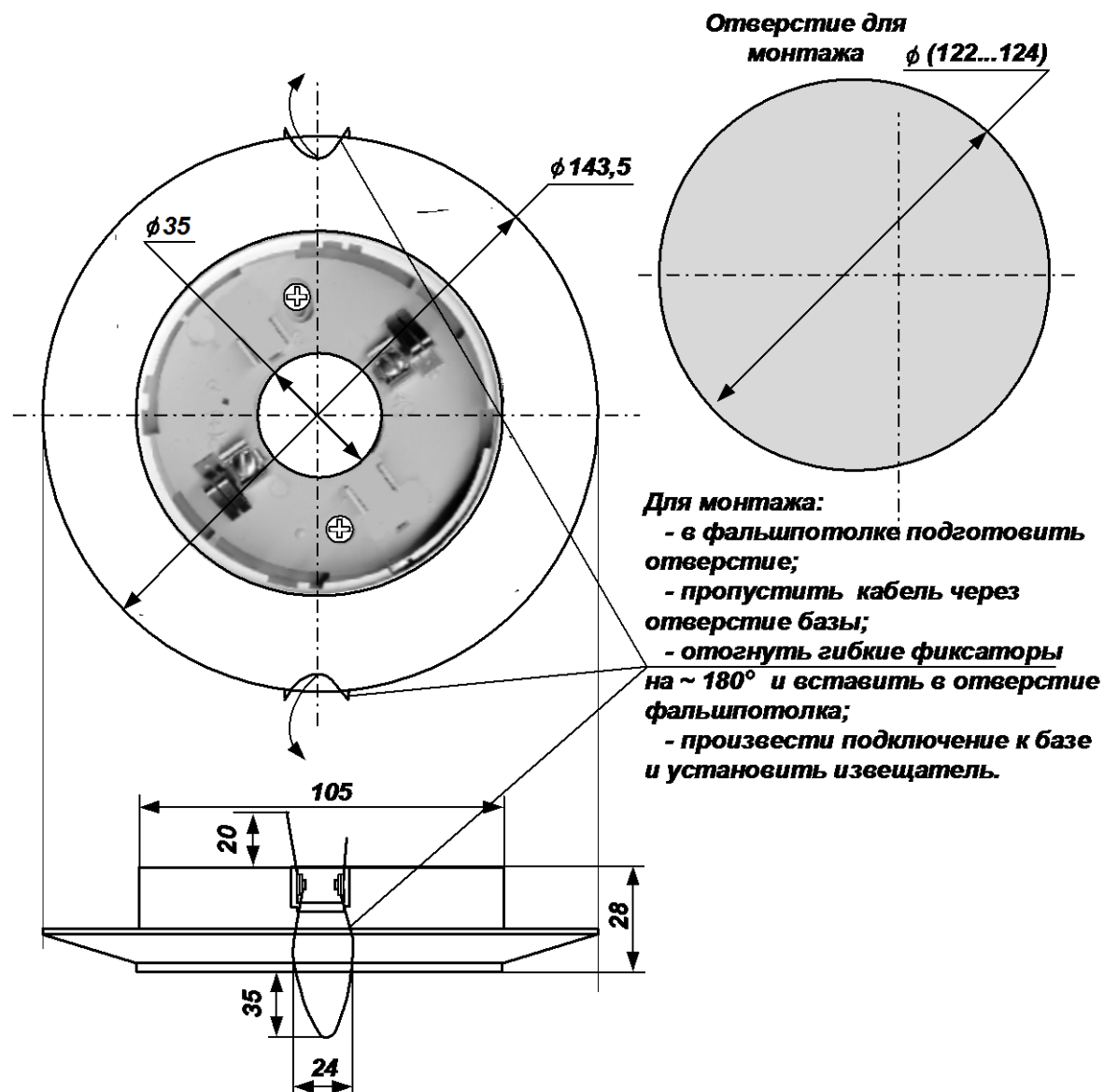
Рис. 4 Основные размеры и отверстие для монтажа базы в исполнении для подвесного потолка
