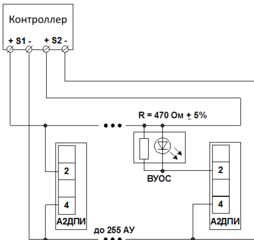
Рис. 5 Подключение А2ДПИ в АШ. Подключение ВУОС.
