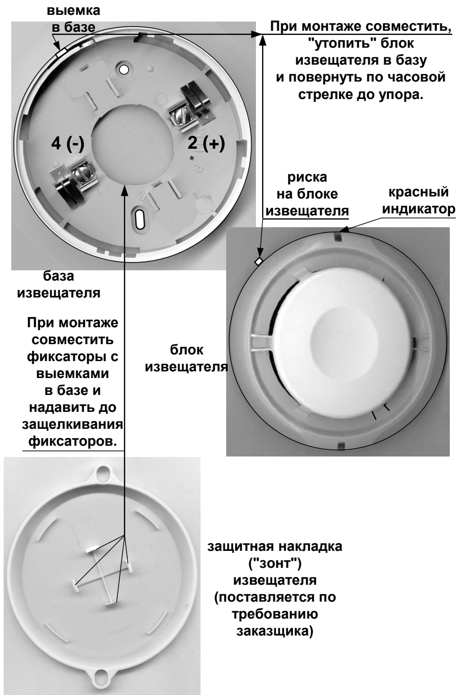
Рис. 2 А2ДПИ. База, блок извещателя, накладка "Зонт"
