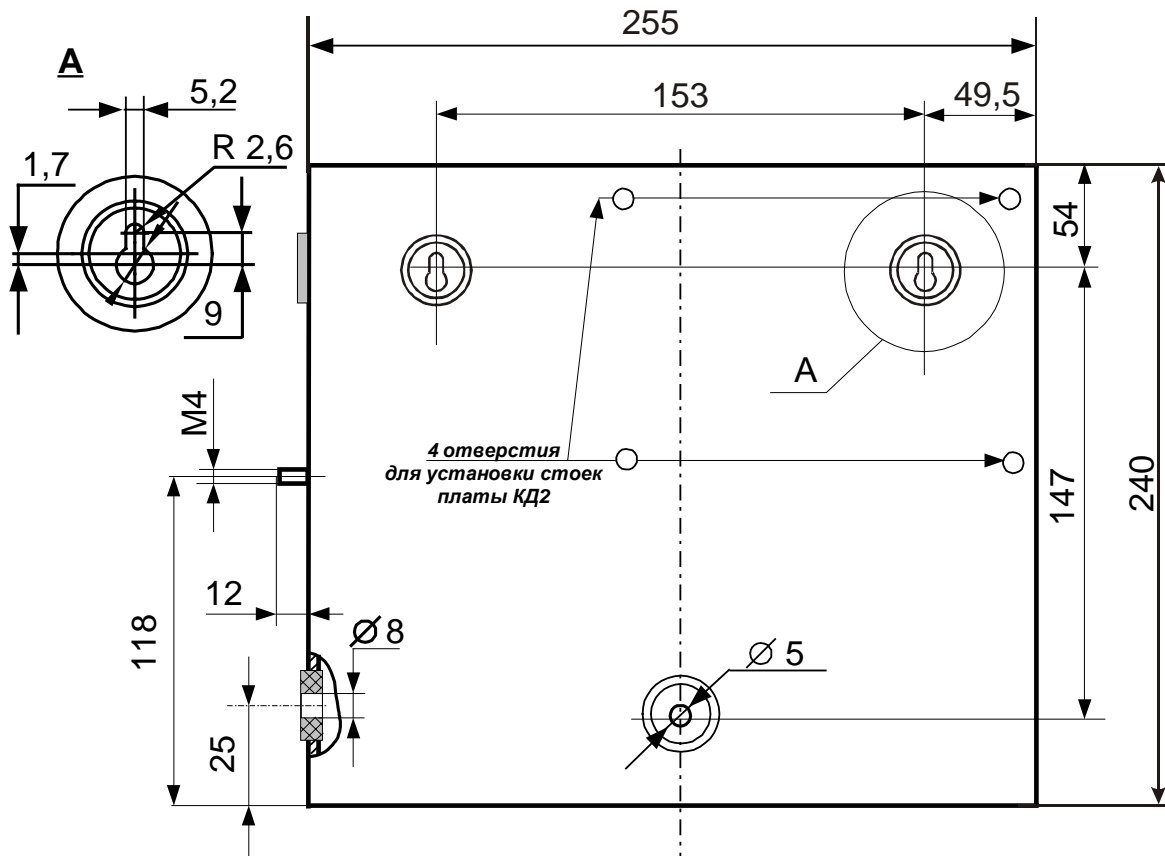
Рис. 11 Габаритные и присоединительные размеры КД2 исп. 1. Вид сзади
