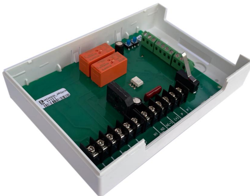
Рис. 1 Внешний вид ИСМ со снятой крышкой
