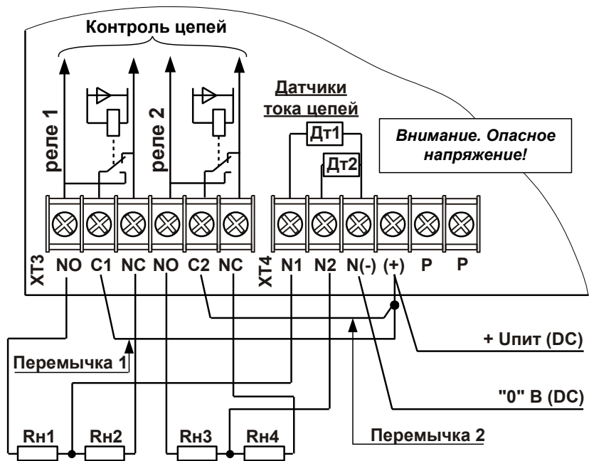
б) Подключение нагрузок к сети постоянного тока =Упит, Упит - (11 ... 50) В, I н ≤ 3 А
