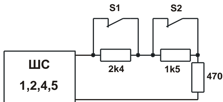
Рис. 10 Последовательное подключение 2 извещателей с НЗ контактами
