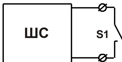
Рис. 18 Подключение извещателя с НР контактами без контроля целостности линии связи
