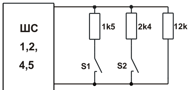
Рис. 11 Параллельное подключение 2 извещателей с НР контактами
