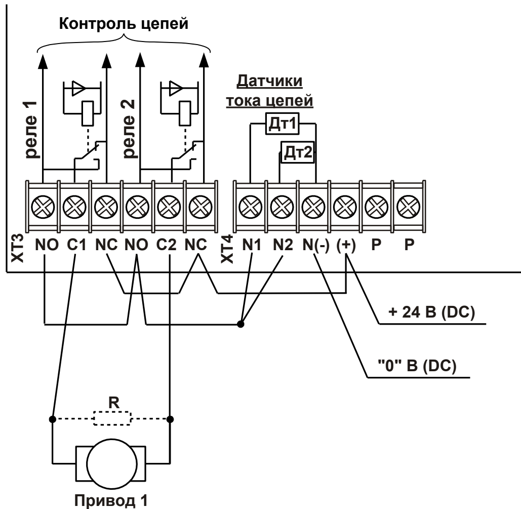
Рис. 9 Подключение реверсивного привода постоянного тока с переполюсовкой
