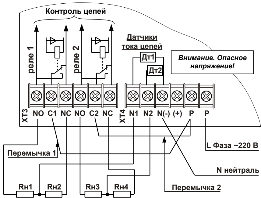
а) Подключение нагрузок к сети переменного тока ~220 В, 50 Гц, ~U - (160 ... 260) В, I н ≤ 3 А
