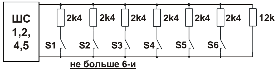
Рис. 15 Параллельное подключение нескольких НР извещателей
