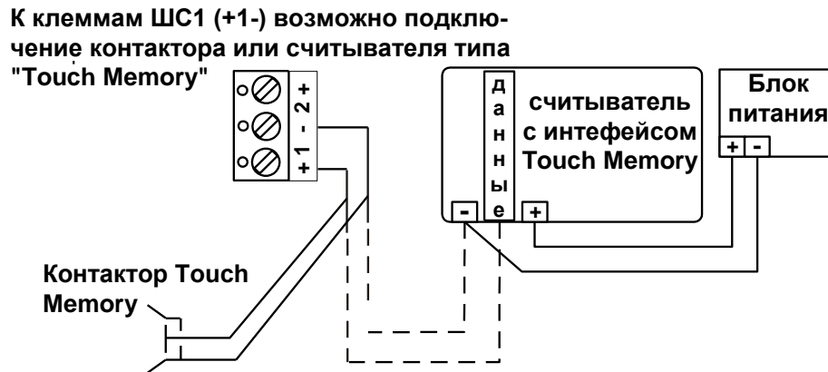
Рис. 21 Подключение контактора (считывателя – пунктиром) "Touch Memory"
