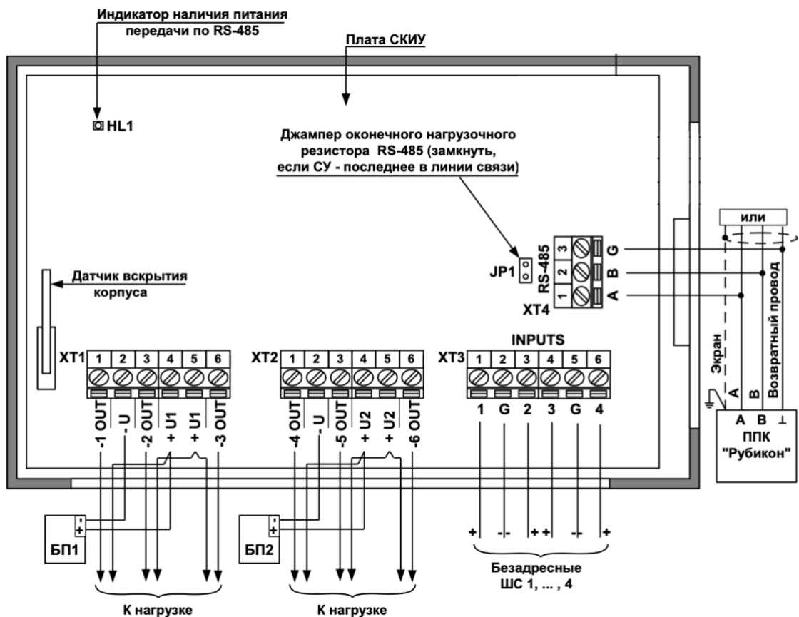
Рис. 1 СКИУ-06. Расположение элементов. Подключение.
