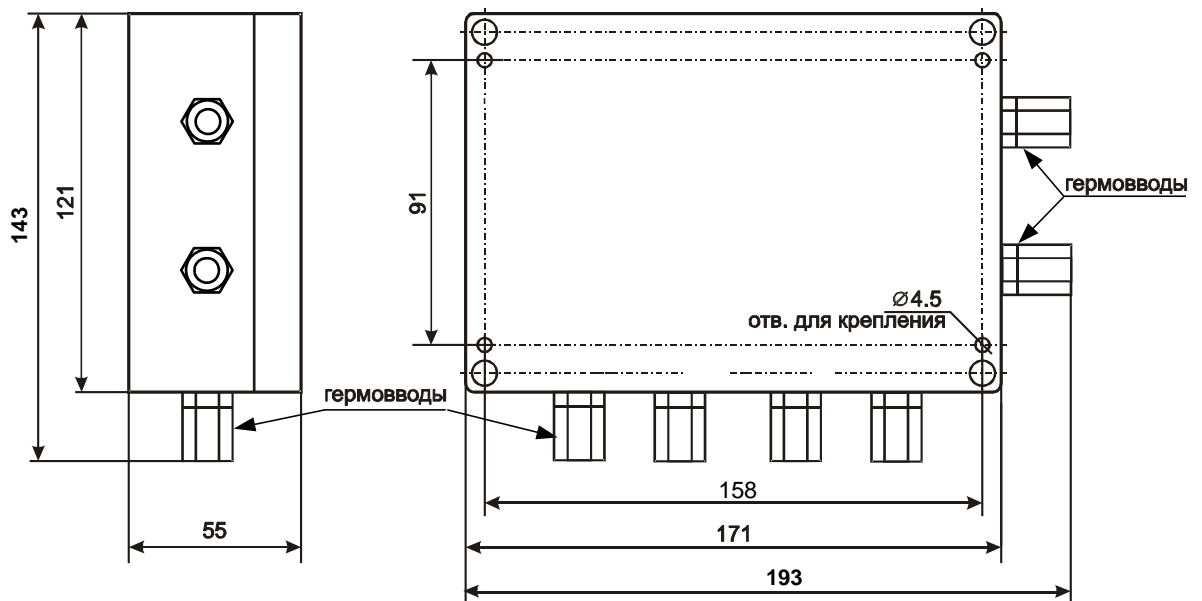
Рис. 3 Внешний вид, габаритные и присоединительные размеры (исполнение IP65)
