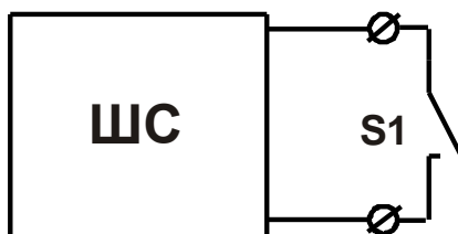
Рис. Схема 4. Подключение извещателя (датчика) с НР контактами без контроля целостности линии связи.
