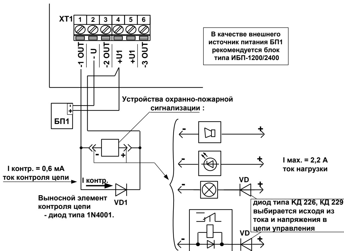
Рис. 4 Подключение исполнительных устройств
