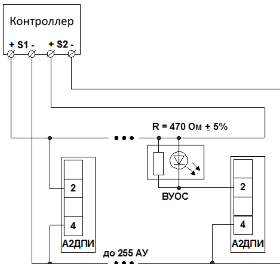
Рисунок 5 – Подключение А2ДПИ в АШ. Подключение ВУОС
