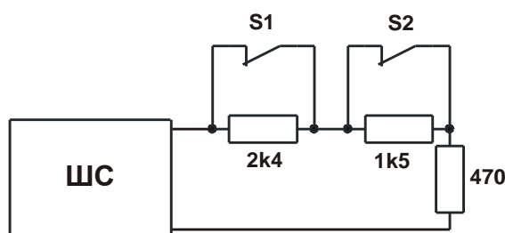
Рисунок-схема 1 – Последовательное подключение двух извещателей с НЗ контактами
