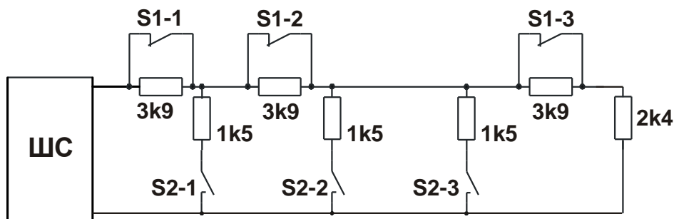
Рисунок-схема 9 – Параллельно-последовательное подключение и НЗ, и НР извещателей
