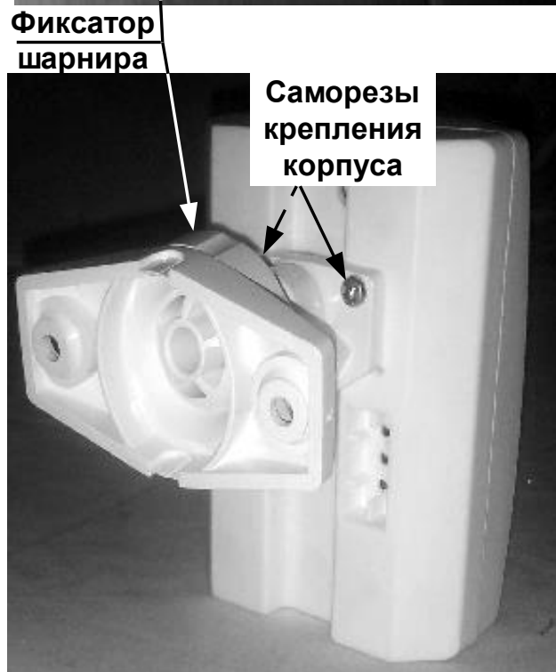
б) Шарнирный кронштейн с фиксацией
