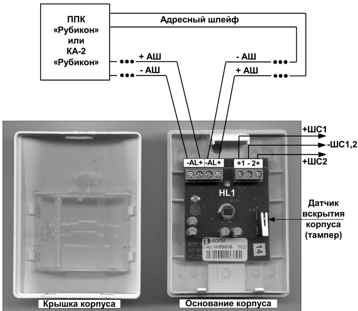
Рисунок 2 – Конструкция, подключение АОПИ
