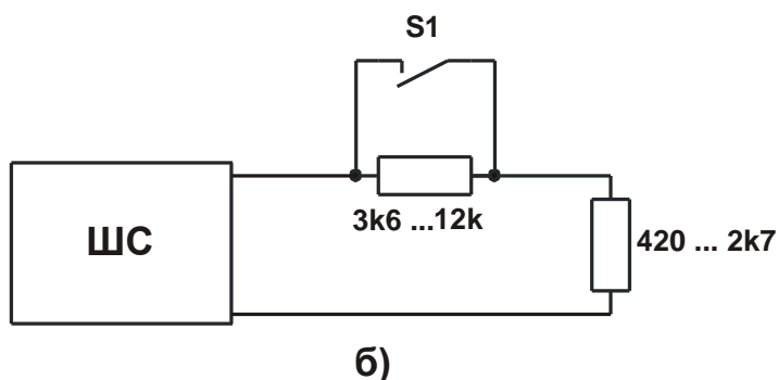
Рисунок-схема 4 – а) параллельное подключение 1-го извещателя с НР контактами; б) последовательное подключение 1-го извещателя с НР контактами
