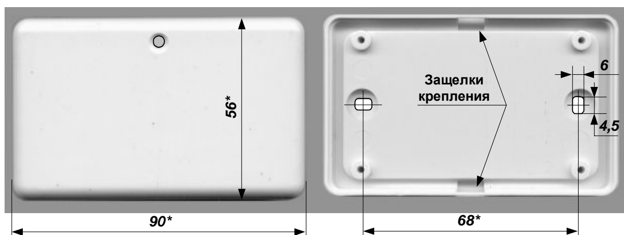
Рис. 2 Габаритные и присоединительные размеры корпуса ИСМ
